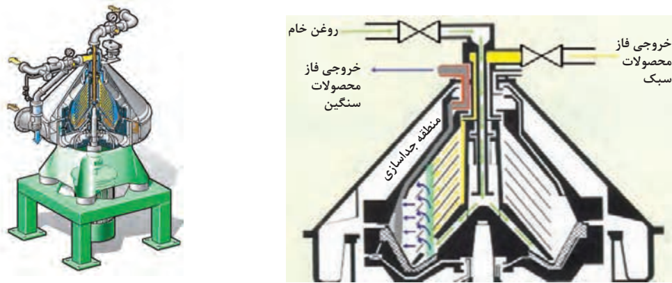
شکل ۷- شماتیک سانتریفیوژ
